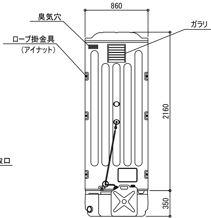
裏面図
