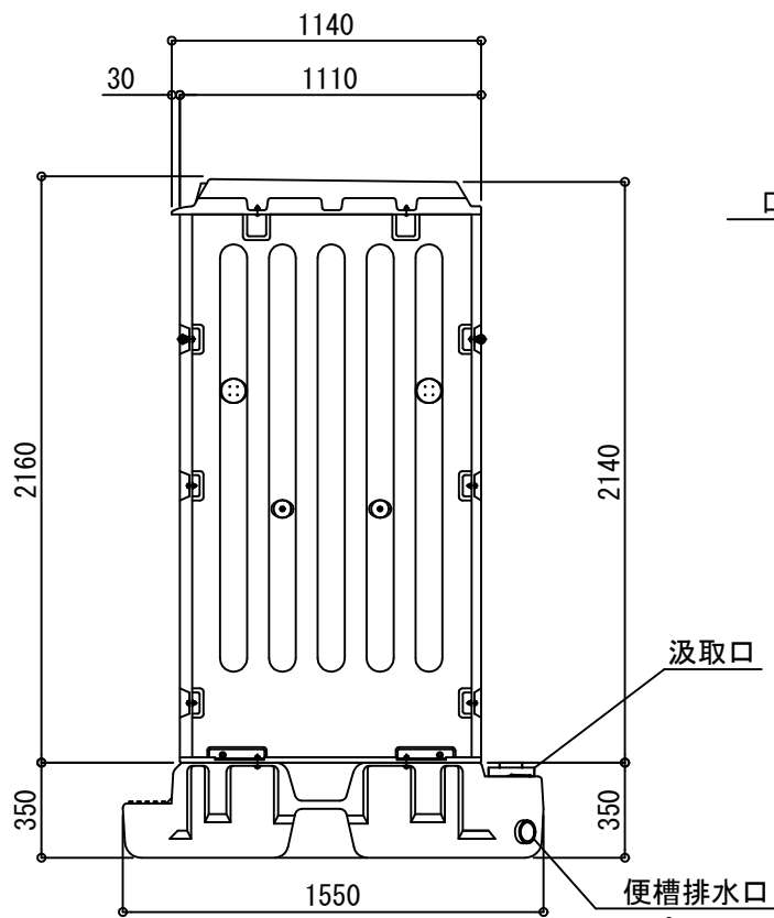
側面図
