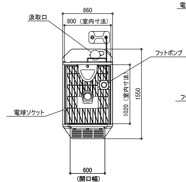
平面図
