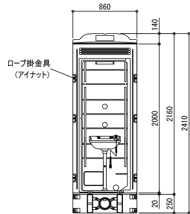
正面図
