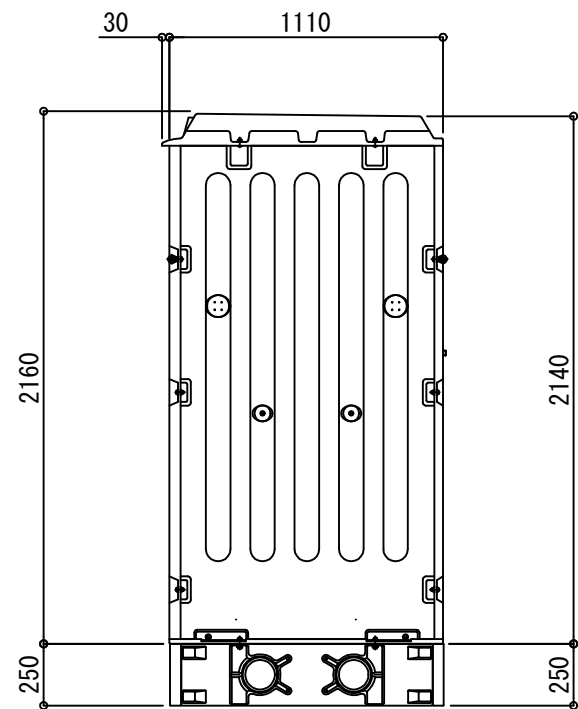
側面図
