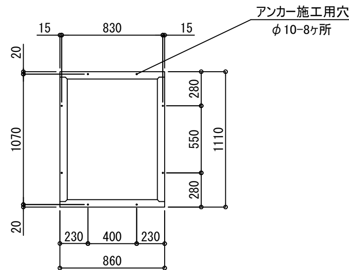
床伏図
